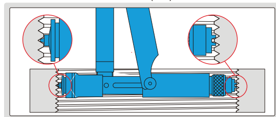
测量原理(C型)
