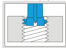
测量原理(A型)
